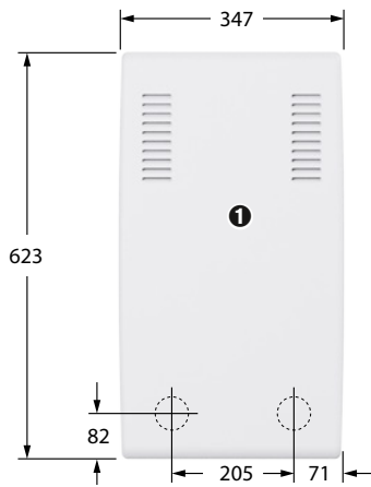
Frontansicht (Längenangaben in mm)
