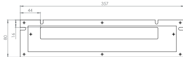
RÖPS 01 - Putzschutz Front- und Seitenansicht
