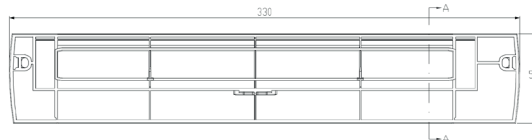
ROLE 01 - Luftmengenerhöhung Front- und Seitenansicht
