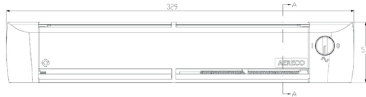
ZUROH 110 Front- und Seitenansicht
