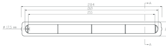
ROLK 01 - Luftkanal Front- und Seitenansicht
