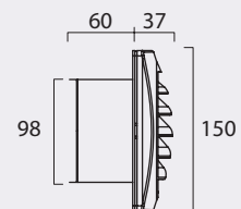
Seitenansicht
